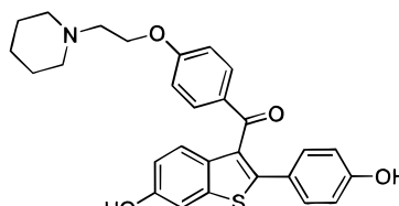
Raloxifene
